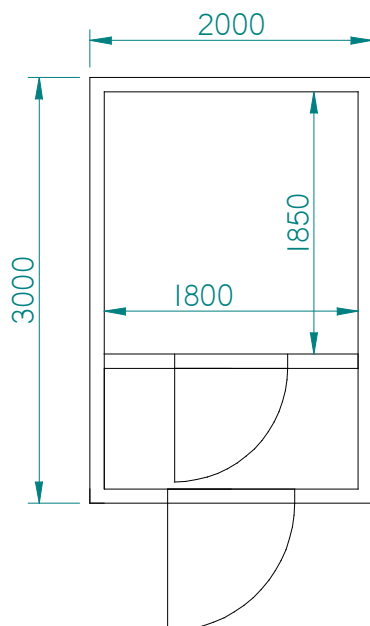
Rys. nr 1 Schemat chłodni
